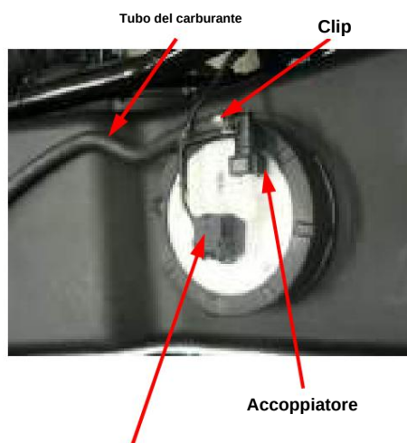
Indicatore del connettore, serbatoio del carburante
